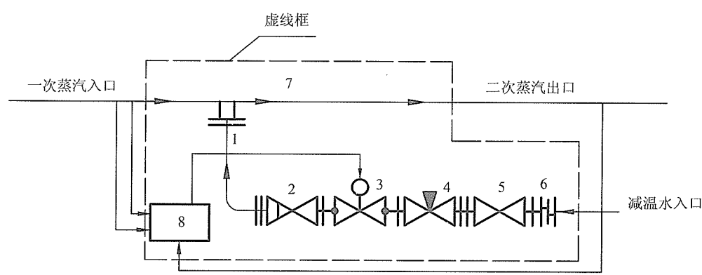
图 B.2 典型的减温减压分体结构系统图例
